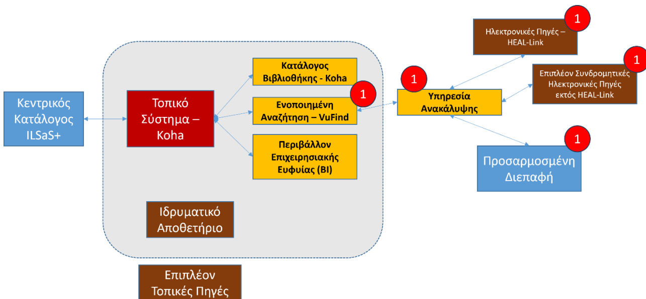
Εικόνα 1. Αρχιτεκτονική πρώτου σεναρίου εγκατάστασης
